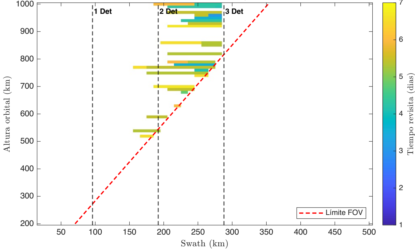
Tiempo Revisita - 2 Satelite(s); 2 Telescopio(s): Refractivo; Detector 1 (Blanco: \geq 7 dias)
